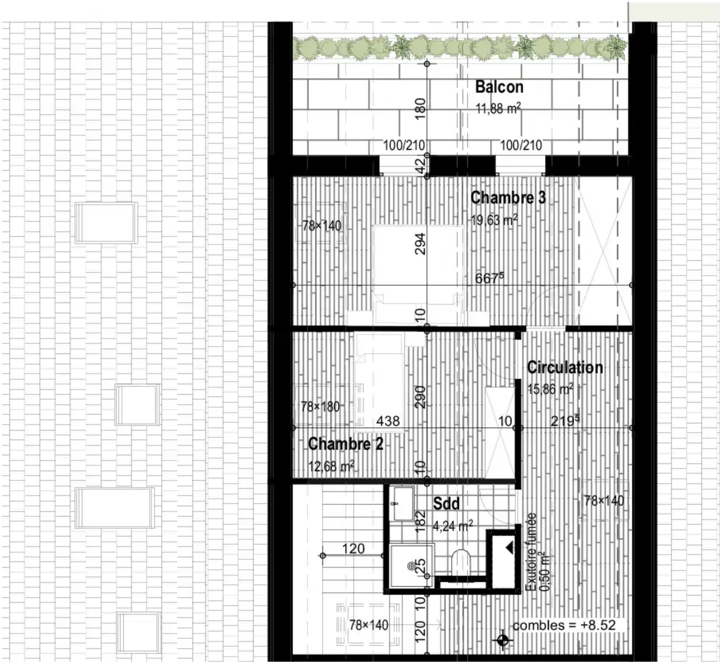
SUR-COMBLES
